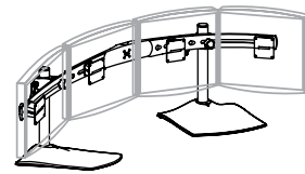
33-284-200、 独立式底座（2个）、 14英寸立杆（2个）、 55英寸横杆、外置立杆夹、 滑动转轴（4个）
